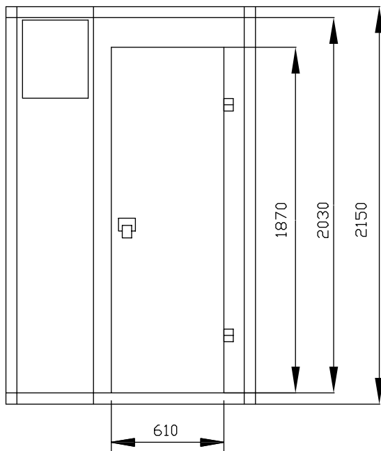
Zij aanzicht
